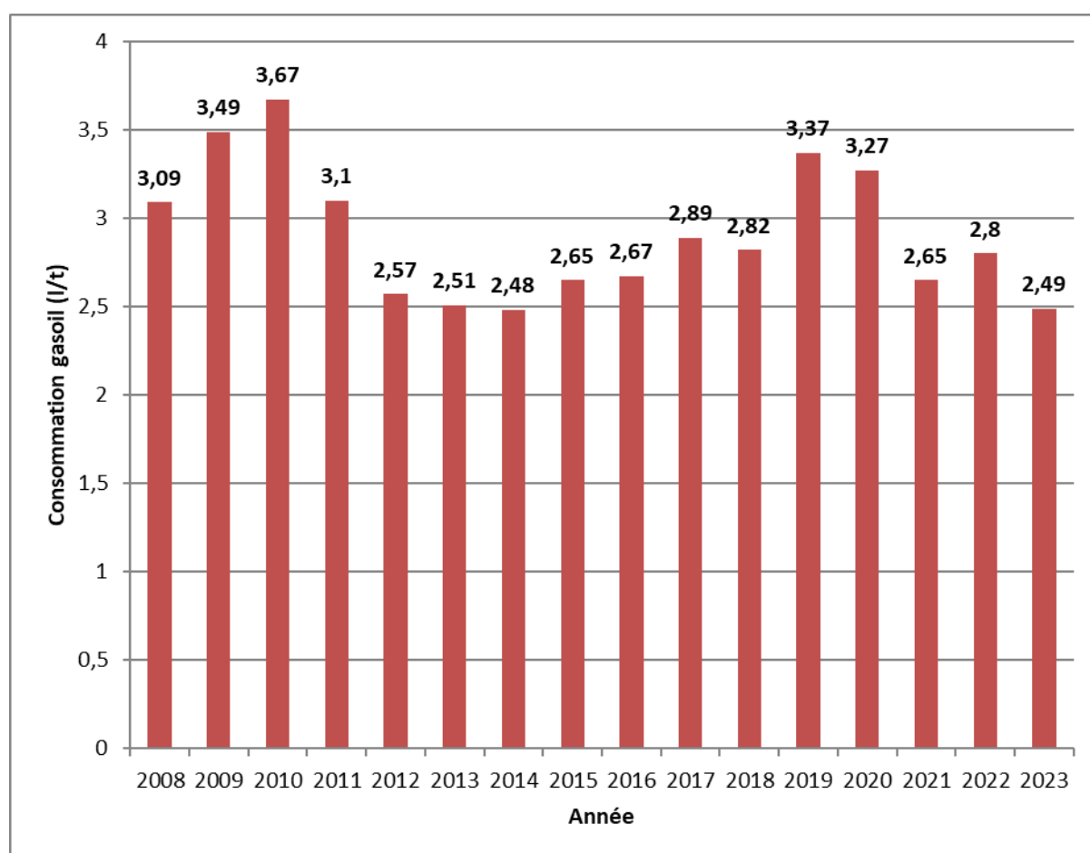
Historique des consommations spécifiques de gasoil
